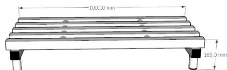
PA500 5kg - 0,10m 3
